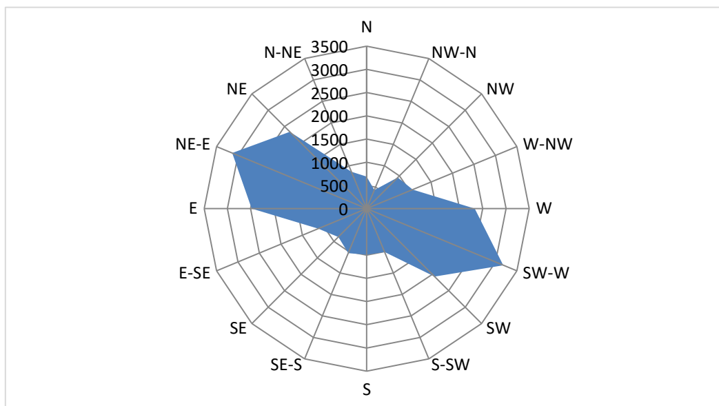
Figura n. 3 – Distribuzione statistica della direzione del vento (Tavazzano con Villavesco)
